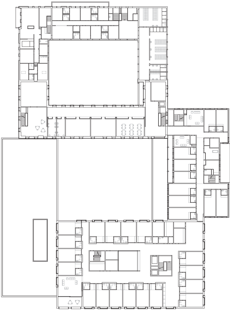
Regelgeschoss, 1:600
